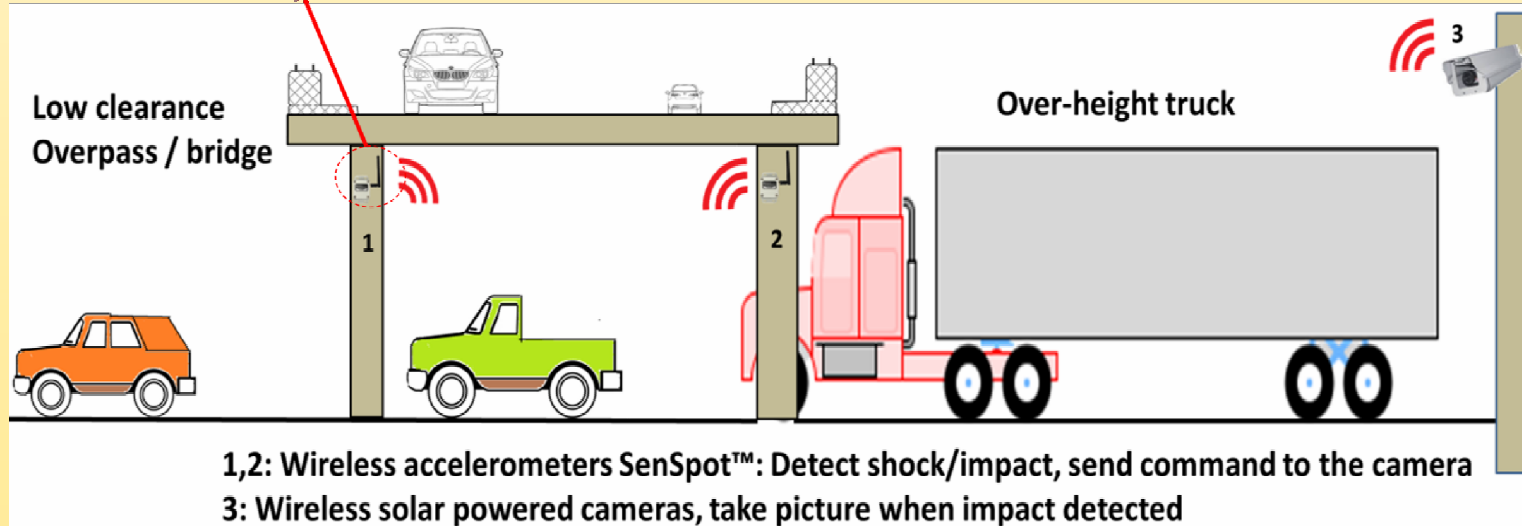
Pristup detekciji sudara vozila koristeći bežični akcelometar i bežičnu solarnu kameru
