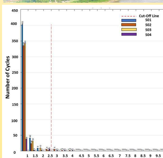
Raspodela frekvencije (histogram) opsega napreznja na bežičnim senzorima napreznja SenSpot u softveru SenScope™
